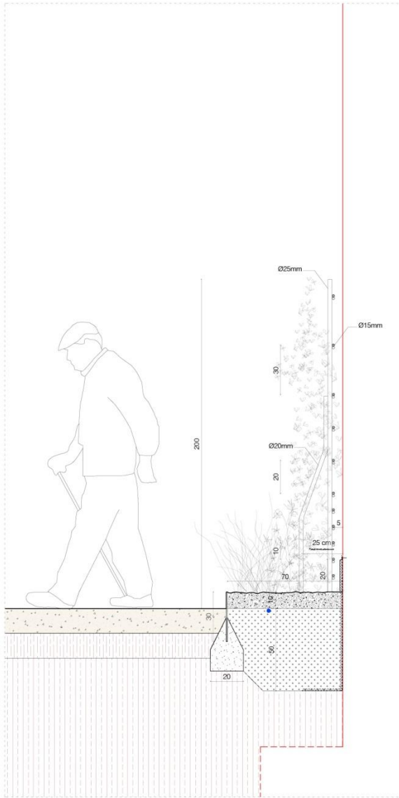
DET 03 e:1/20
