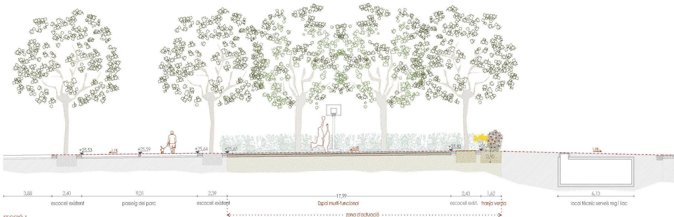
SECCIÓ 1
