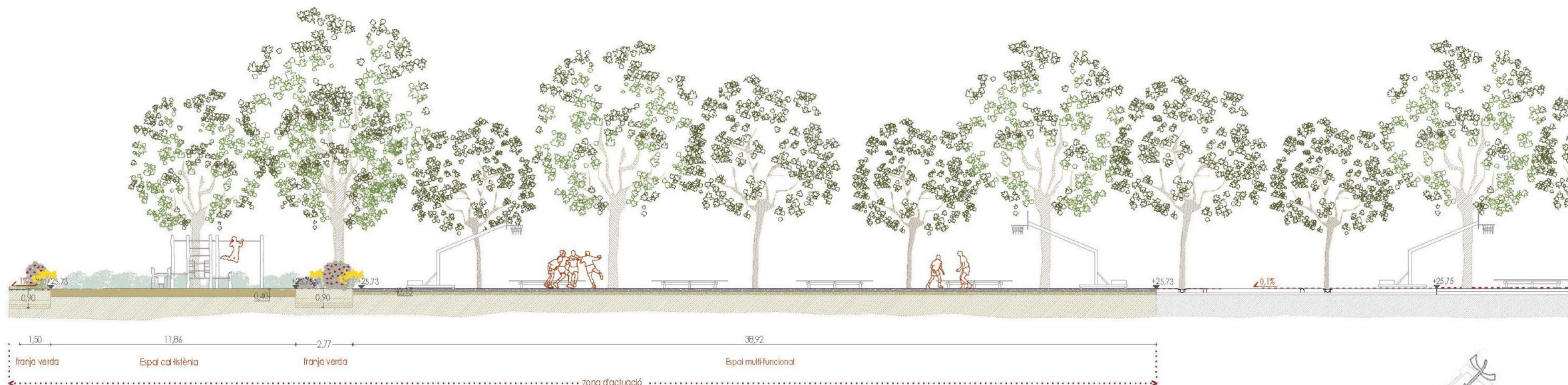
SECCIÓ 7
