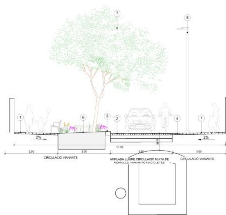
SECCIÓ B-B' ESC. 1/75
