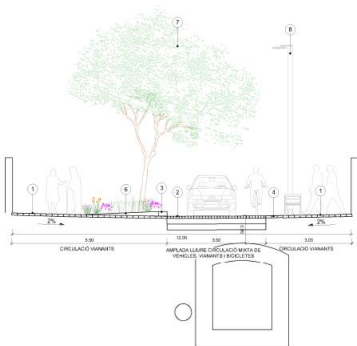
SECCIÓ A-A' ESC. 1/75
