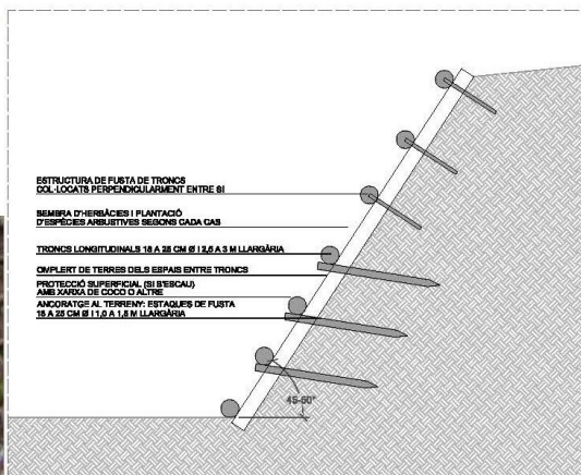
ESQUEMA ENREDAT VII ERC: 1:50 (A1) / 1:100 (A3)
