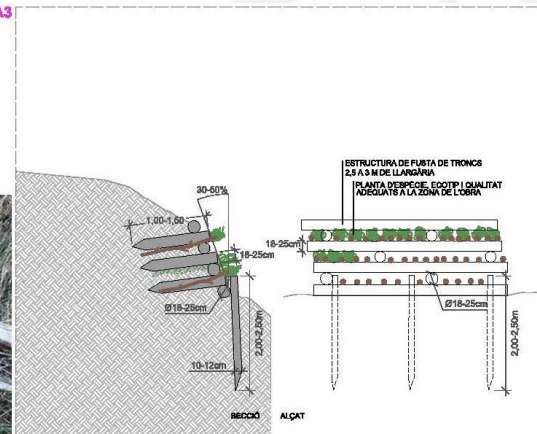
ESQUEMA ENTRAMAT VII ERC: 1:50 (A1) / 1:100 (A3)
