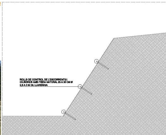
ESQUEMA PEDONA ERC: 1:50 (A1) / 1:100 (A3)
