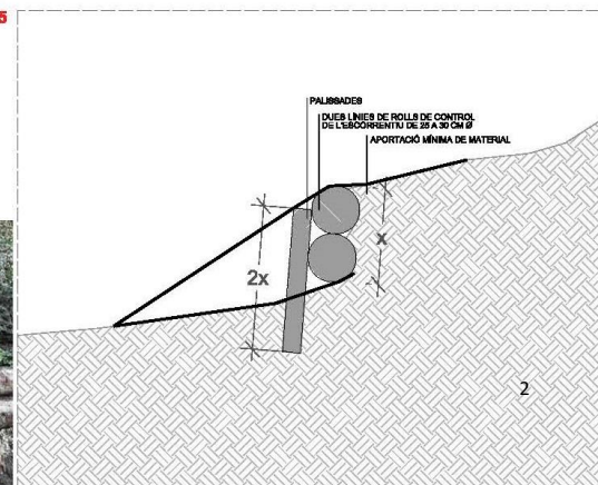
ESQUEMA PALISSADA ERC: 1:25 (A1) / 1:50 (A3)
