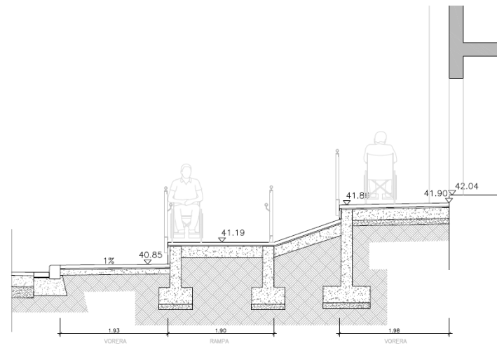
D-D'
