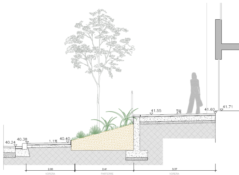
A-A'
