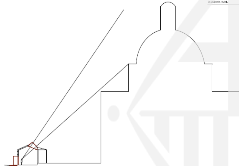
ESQUEMA LLUERNARI AMB VISTES A LA CÚPULA DE SANT ANDREU DEL PALOMAR
