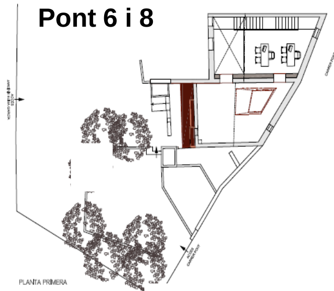
PLANTA PRIMERA
