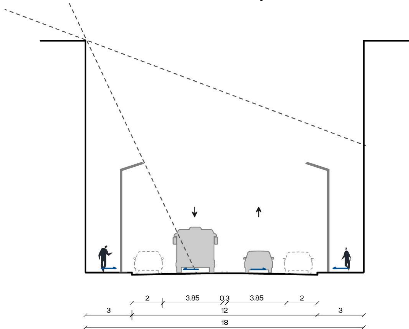
Secció tipus 1
