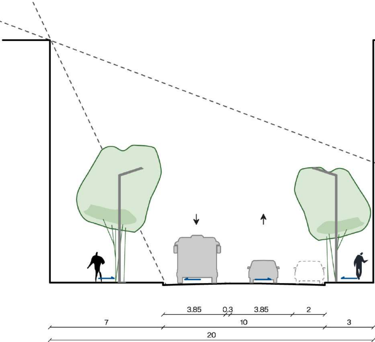
Secció tipus 3
