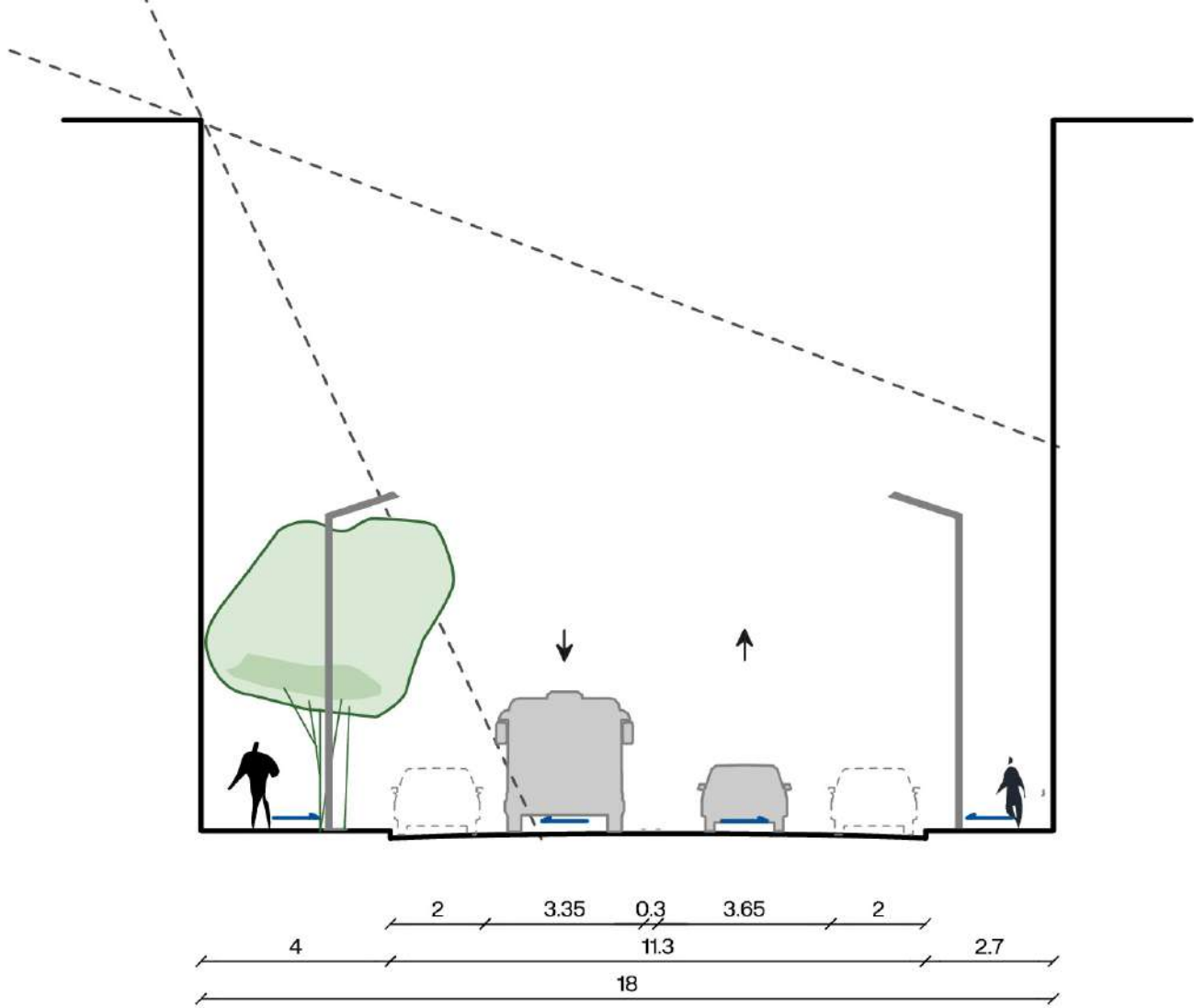
Secció tipus 2
