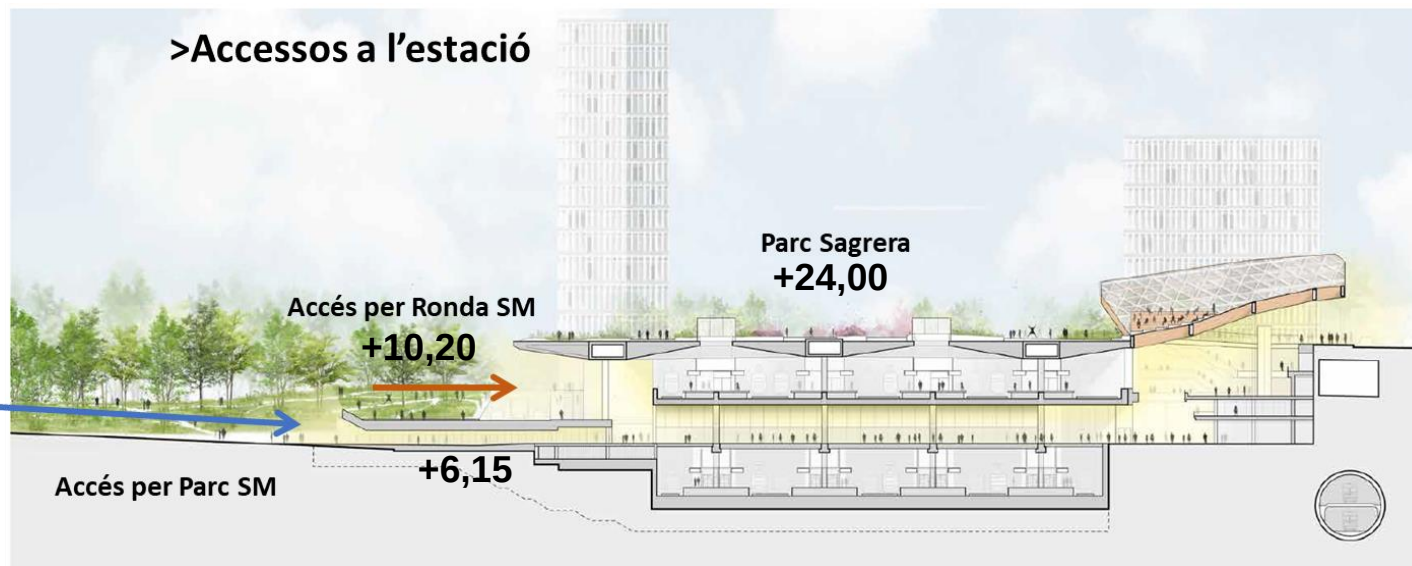
Secció transversal | Porta La Sagrera i porta Sant Martí
