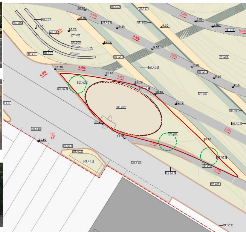
1- SORRA GARBELLADA - paviment no accessible
