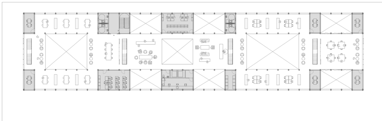
BIBLIOTECA - PLANTA SEGONA
